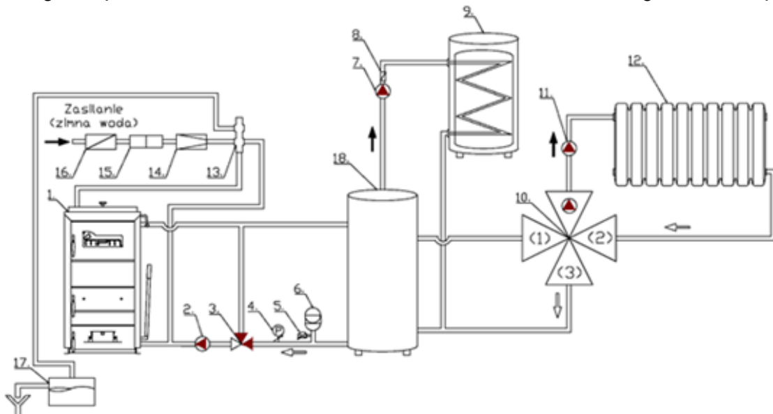
Abbildung 4: Beispielschema für den Anschluss des MPM Wood Plus Holzkessels in einem geschlossenen System.
