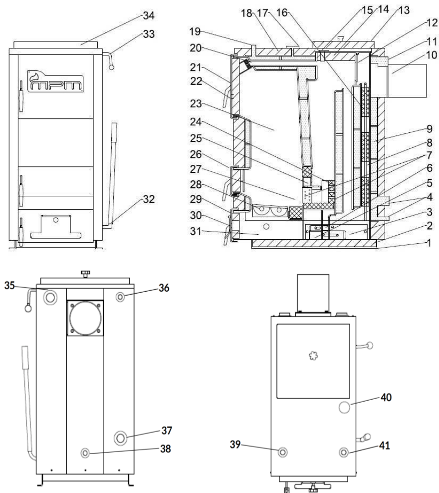
Abbildung 1: Schematische Darstellung eines Seitenladerkessels
