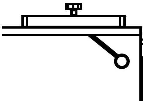
Abbildung 7: Kurzschlussklappenhebel in geöffneter Stellung.
