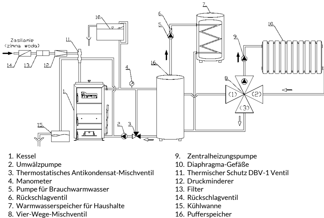
Abbildung 3: Beispielhafte Darstellung des Anschlusses des MPM Wood Plus Holzkessels in einem offenen System.
