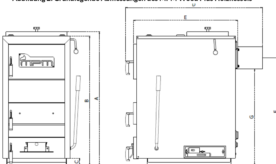
Abbildung 2: Grundlegende Abmessungen des MPM Wood Plus Holzkessels
